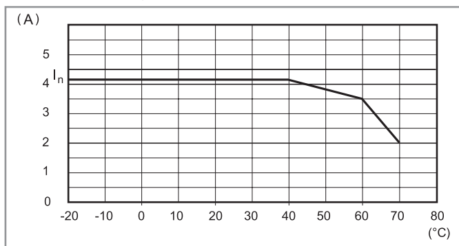
L78-6 Curentul de ieșire vs. temperatura ambiantă (78.50)
