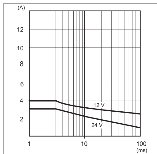
P78-3 Vârful curentului de ieșire vs. timp (78.25)
