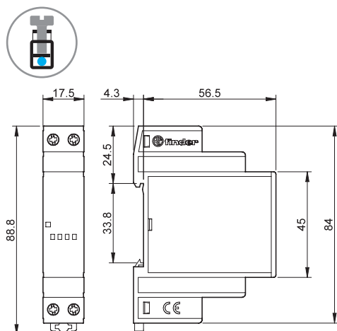
Tipul 78.12 Terminale cu șurub
