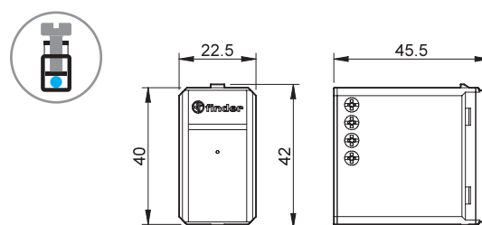
Tipul 15.71 - YESLY Terminal cu șurub
