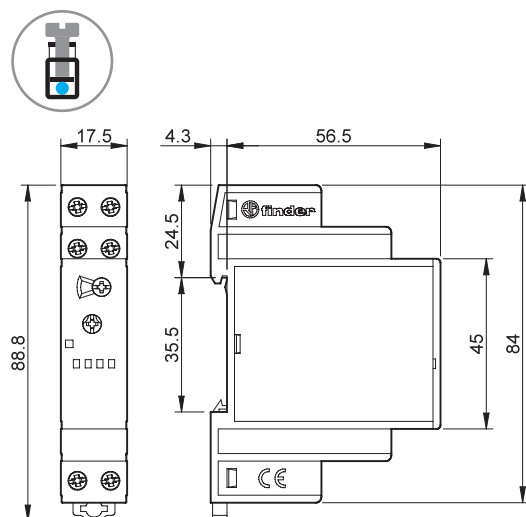
Tipul 13.61.8.230.0000 Terminale cu șurub
