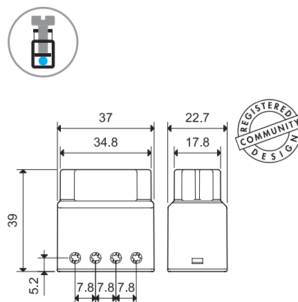
Tipul 13.31/13.91 Terminale cu șurub
