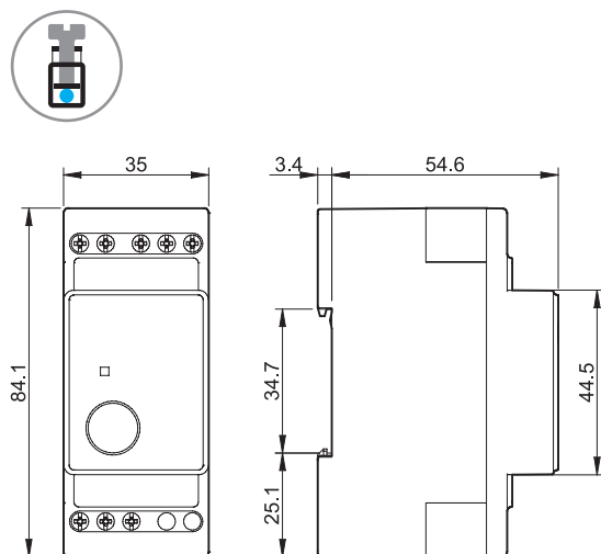
Tipul 13.01 Terminale cu șurub
