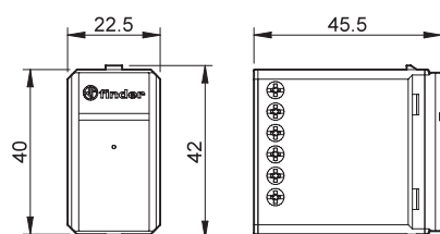
Tipul 13.21.8.230.S000 Terminale cu șurub
