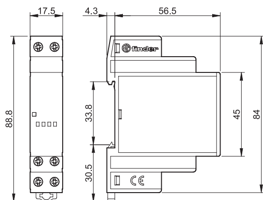
Tipul 13.72 Terminale cu șurub
