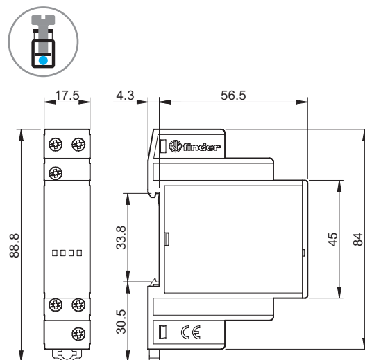
Tipul 13.31/13.91 Terminale cu șurub
