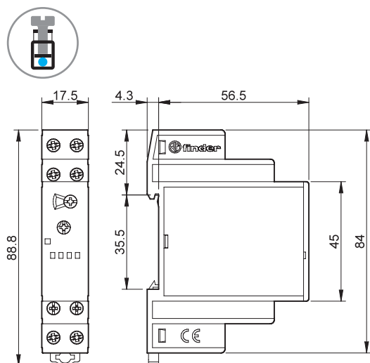
Tipul 13.61.0.024.0000 Terminale cu șurub
