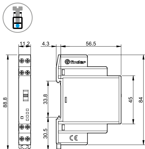
Tipul 19.21 Terminal cu șurub
