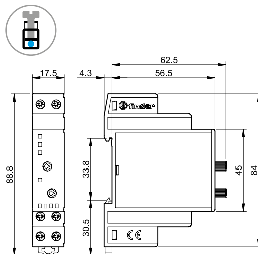
Tipul 19.50 Terminal cu șurub
