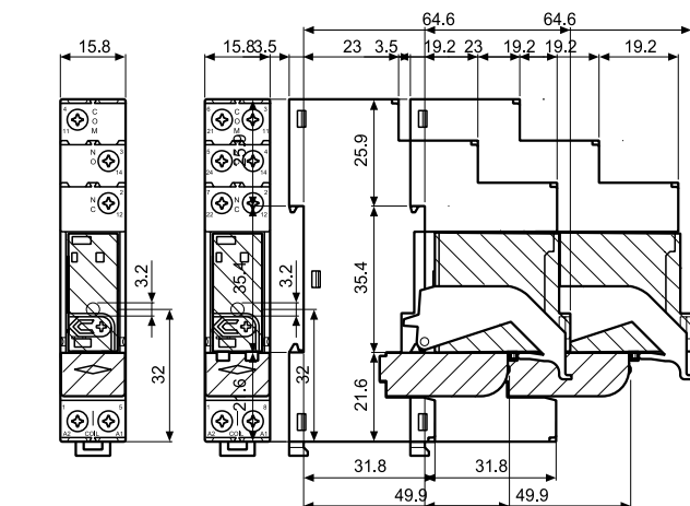
Tipul 4C.01 / 4C.02 Terminale cu șurub
