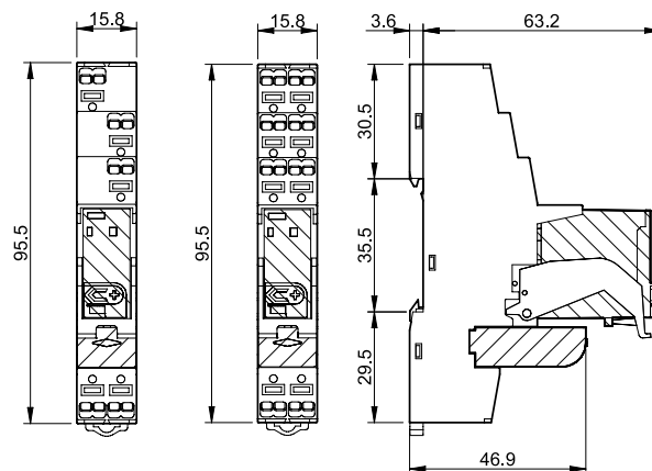
Tipul 4C.P1 / 4C.P2 Terminale „push-in”
