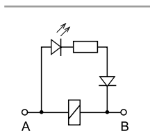
C: Opțiunea 3, 5, 54 LED (C.A.)
