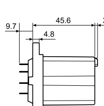
062.10 cu relee
