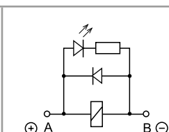
C: Opțiunea 6, 7, 74 LED + diodă (C.C., polaritate pozitivă la pinul A/A1)
