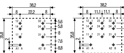
62.22 Vedere de jos (pe partea pinilor)
