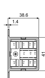
062.60 cu relee
