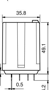
Tipul 62.3x
