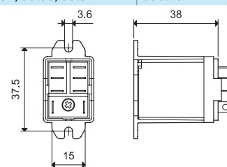
056.25 cu releu
