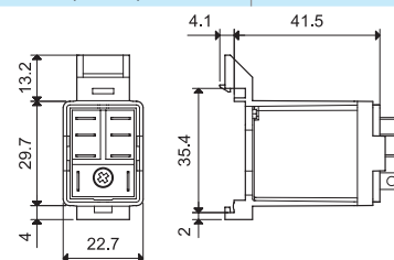
056.27 cu releu
