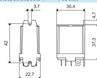
056.26 cu releu
