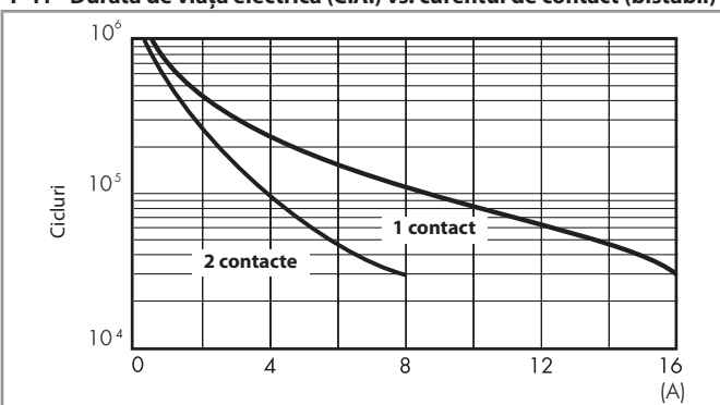
F 41 - Durata de viață electrică (C.A.) vs. curentul de contact (bistabil)
