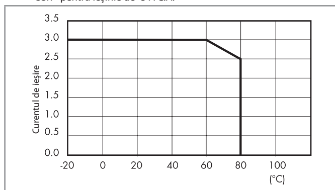
L 41 - Curentul de ieșire vs. temperatura ambiantă SSR - pentru ieșirile de -3 A C.A.
