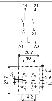
56.42-0300 Vedere de jos (pe partea pinilor)
